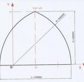
ARCO A SESTO ACUTO
