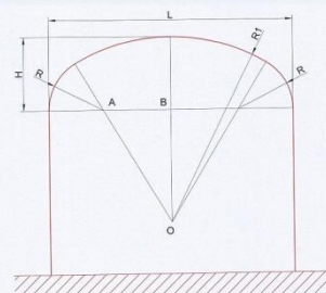
ARCO A TRE CENTRI
